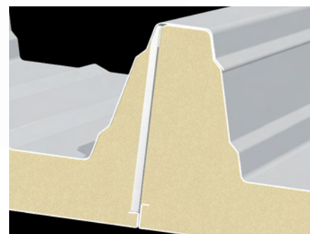
PARTICOLARE DEL GIUNTO
